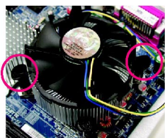
図 3 ヒートシンクをCPUの上へのせ、プッシュピンがマザーボード上のピン穴に向いているか確認します。プッシュピンを斜めに押し下げます。
