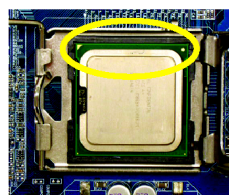
図 3 CPU ソケット端に位置する小さな金色の三角形に注目します。CPU の刻み目のある角を三角形に合わせ、CPU を静かに
